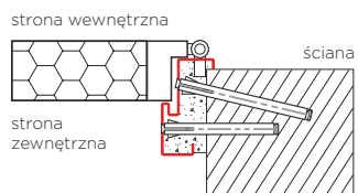
drzwi wewnętrzne otwierane do wewnątrz ościeżnica PU/UNI56
